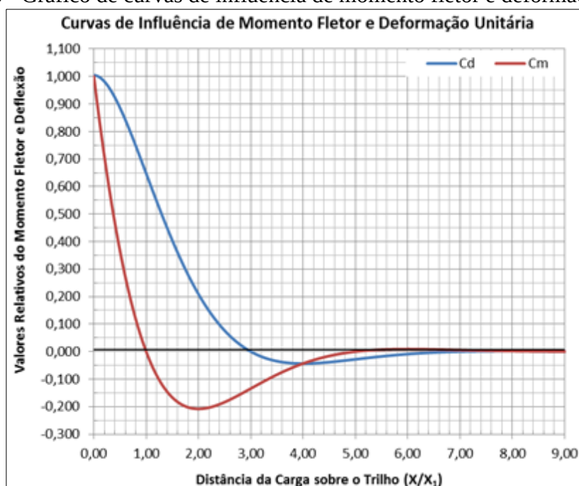
Figura 6 - Gráfico de curvas de influência de momento fletor e deformação unitária
